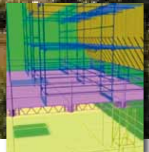
Los diseños fabricados a la medida para andamios Systems y/o QuikDeck en una caldera permiten el acceso fácil.
